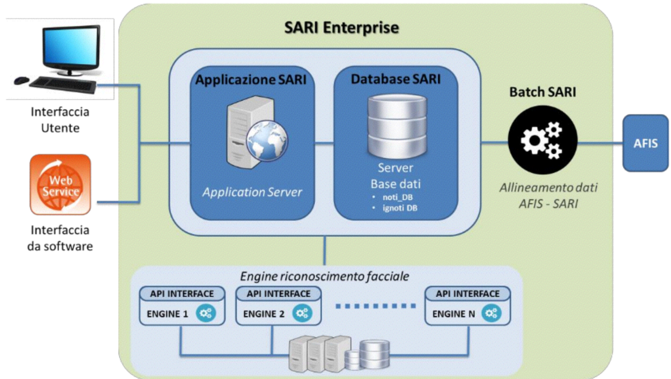
Figura 1-Architettura logica Sistema Enterprise
